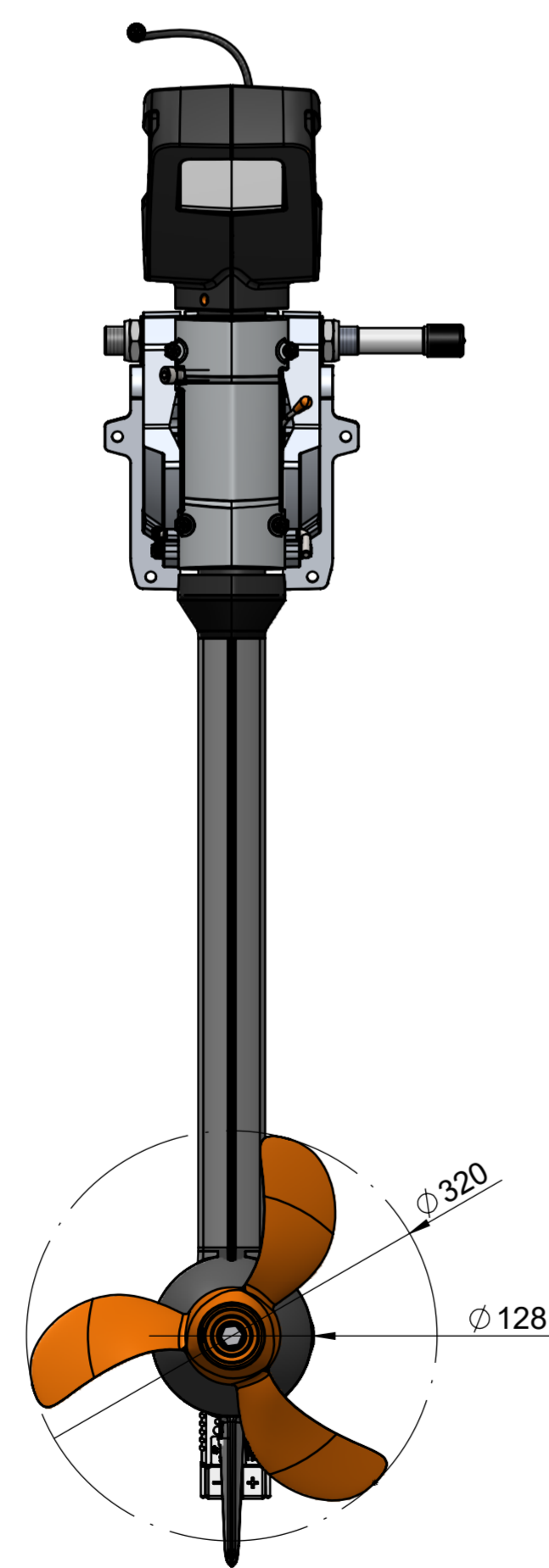
Propeller B 12 x 10,5 WDR
