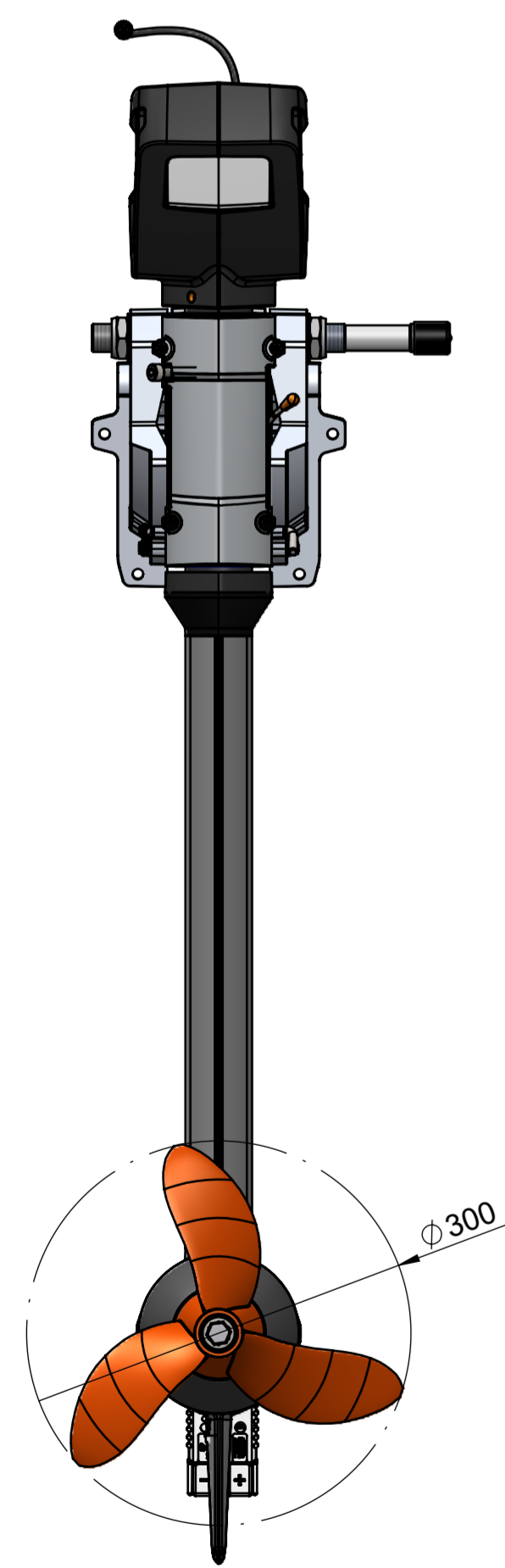
Propeller B 12,5 x 17 HSP
